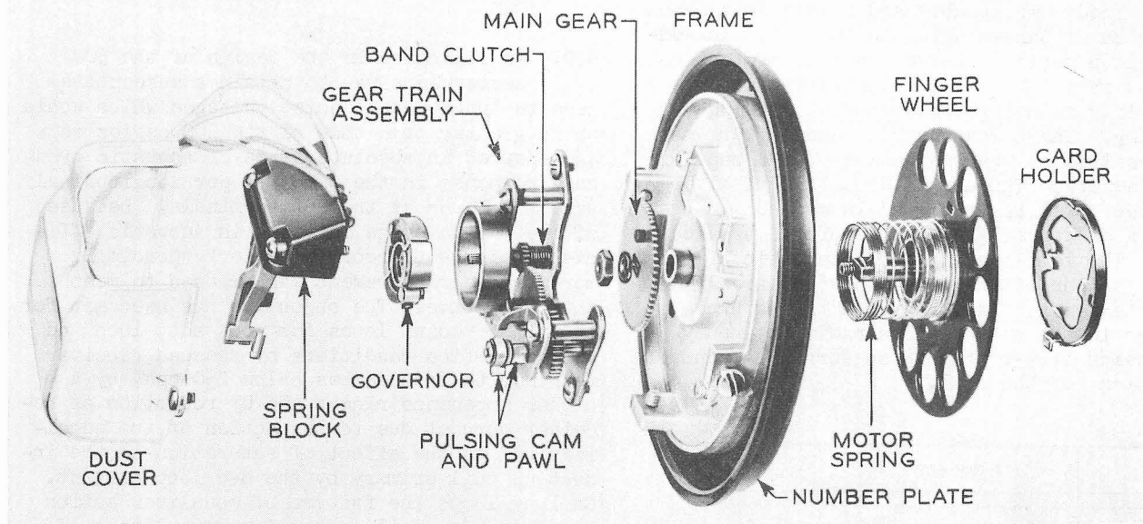
Fig. 11 - 7A-3 Dial
