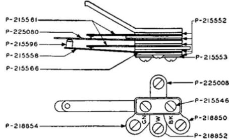
RIGHT PER A-148808 FIG. 2
