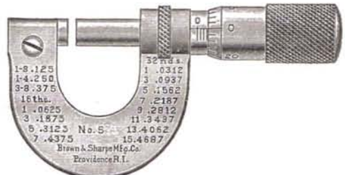
Micrometer Caliper
