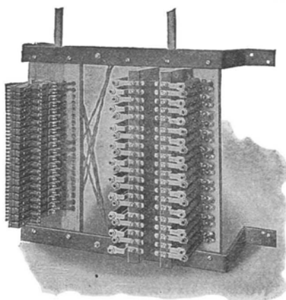
No. 1431-A —20-Line Main
