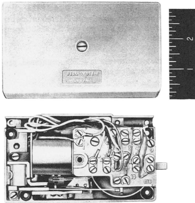
Fig. 7 — E1B Ringer
