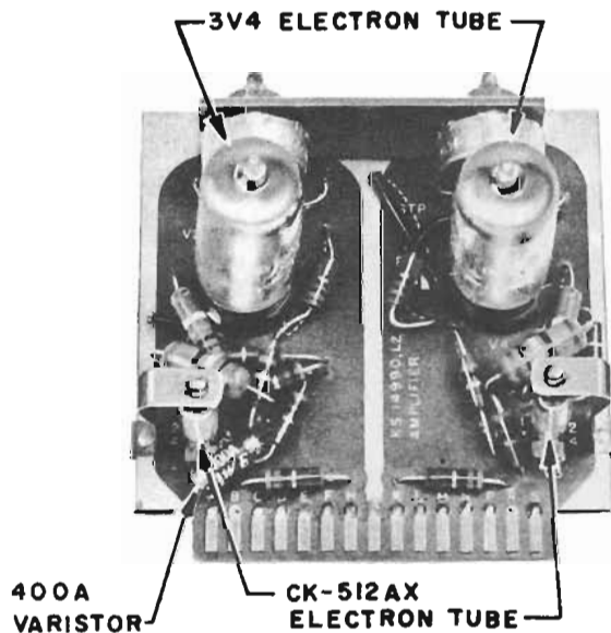
Fig. 7 — KS-14990, List 2 Amplifier
