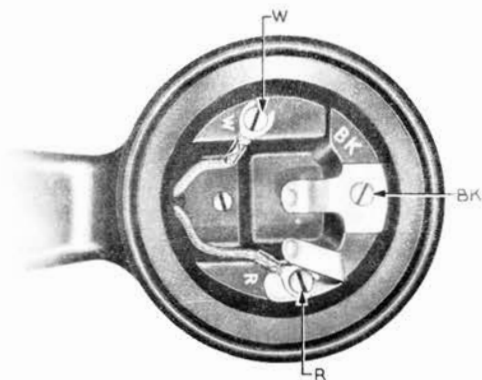
FIG. 3—F4-TYPE HANDSET
