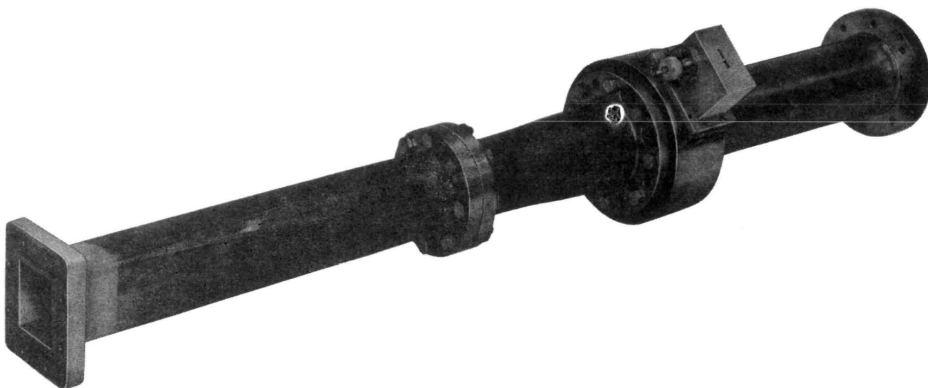
Fig. 1 — 21A Coupler
