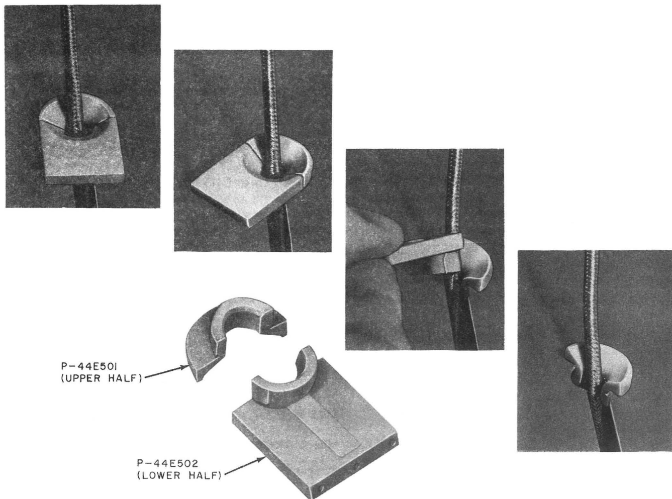
Fig. 3—Removal of Handset Cord Grommet
