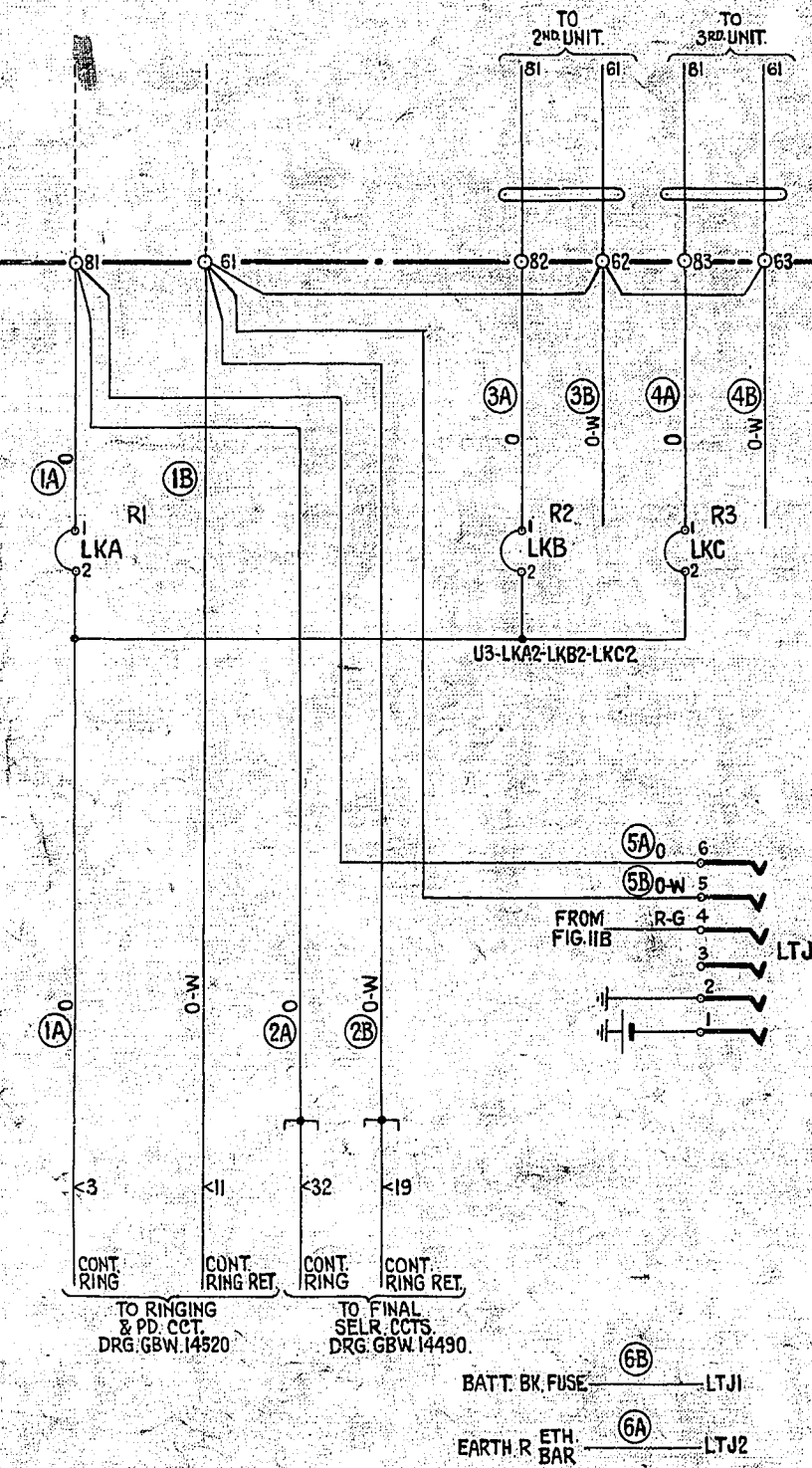
FIG. 9B 1 PER RACK.
