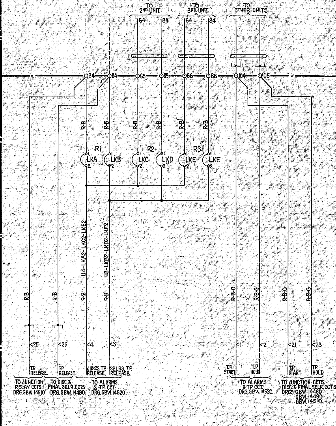
FIG. 10B 1 PER RACK.
