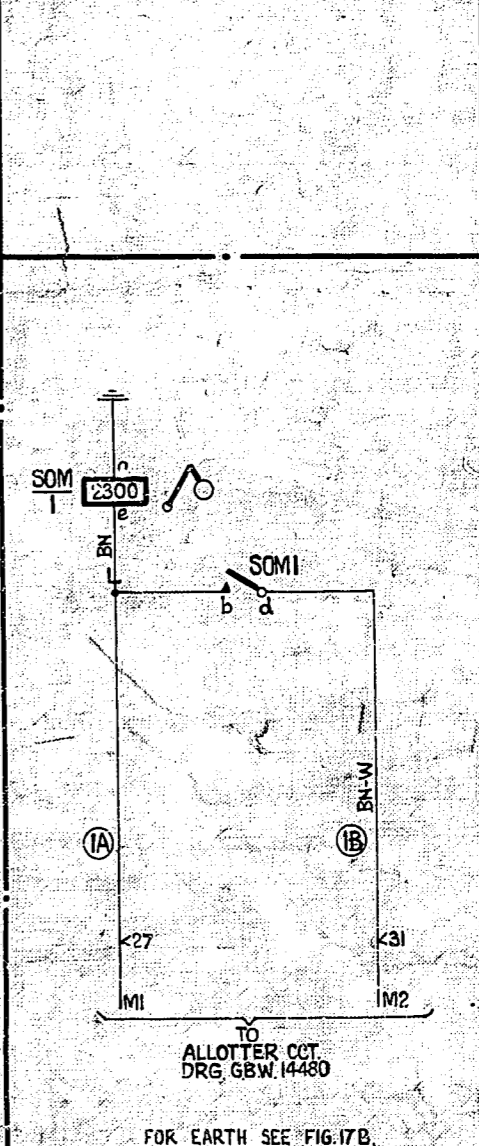
FIG.18B 1 PER RACK
