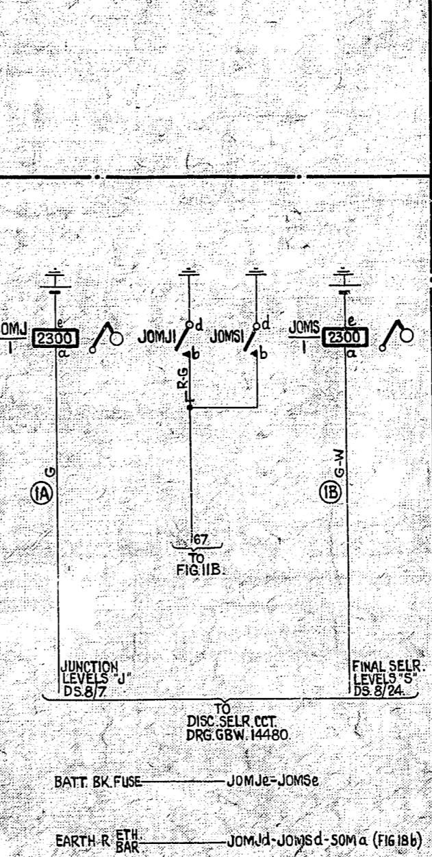
FIG.18B 1 PER RACK
