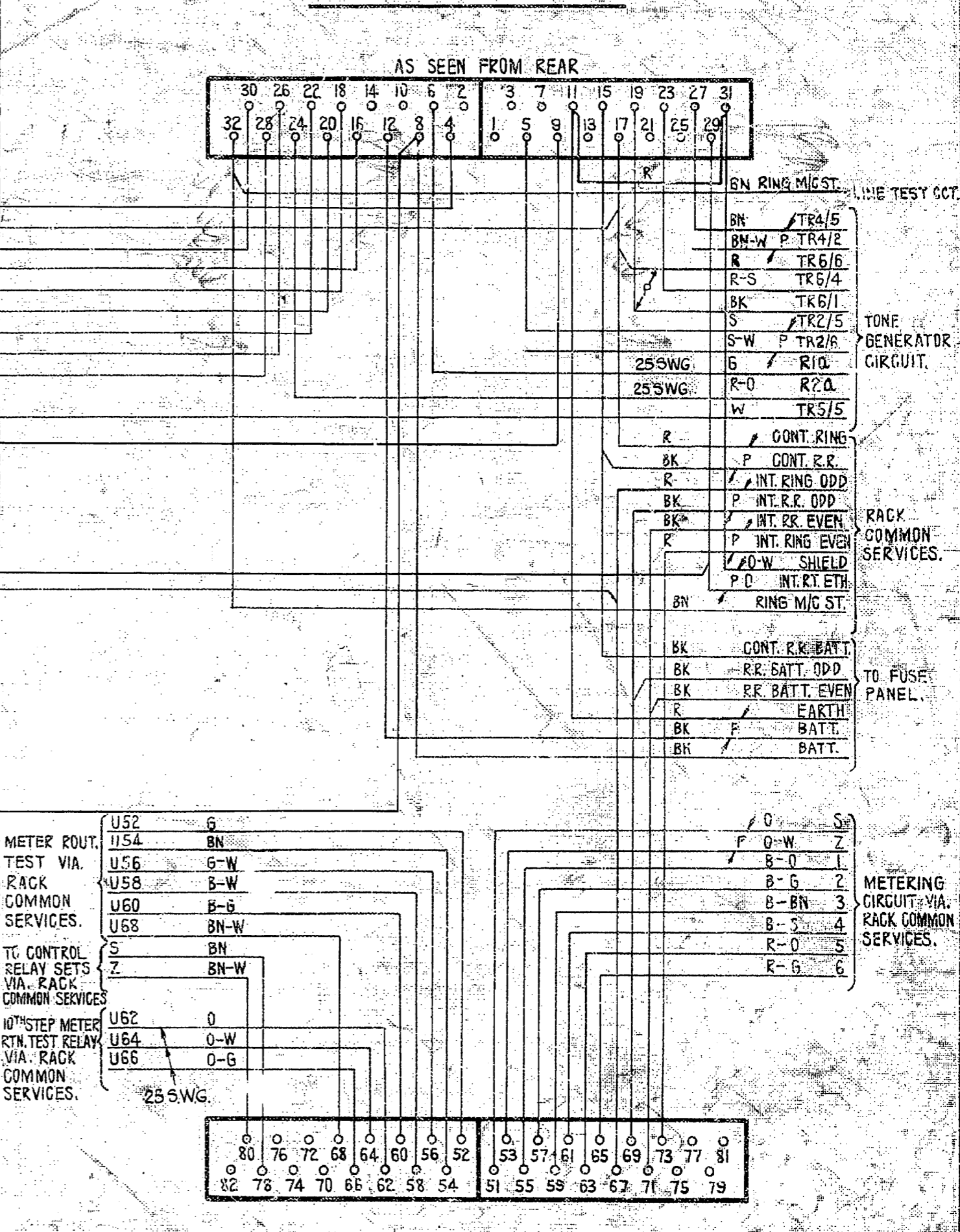
FIG. 2 RINGING METER PULSE C.C.T.
