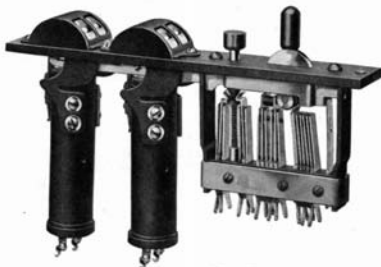
Fig. 15—No. 169 Type Key
