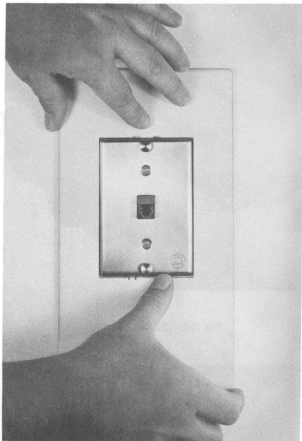
Fig. 16—191-Type Backboard
