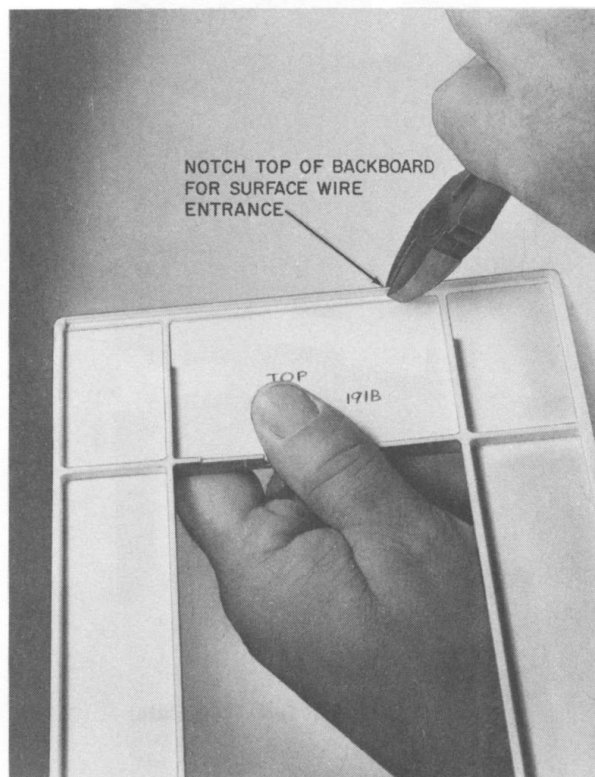
Fig. 16—191-Type Backboard
