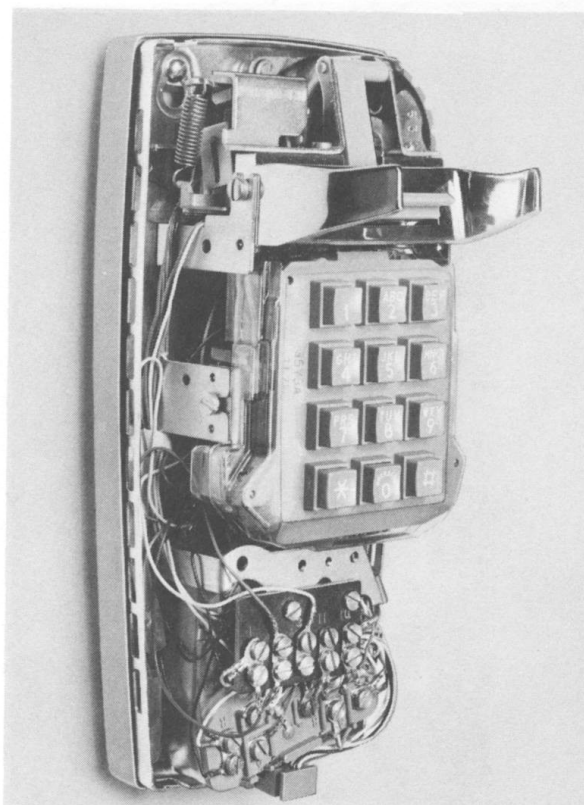
Fig. 33—2554B2P Telephone Set Base
