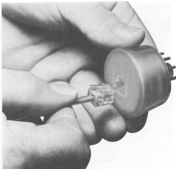
Fig. 21—224A Adapter
