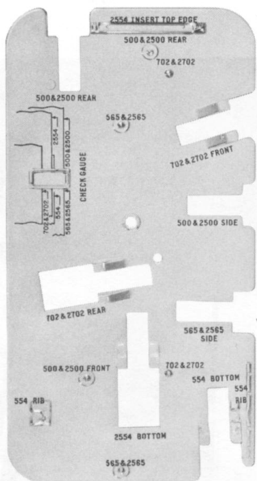
Fig. 19—799A Tool (Template)
