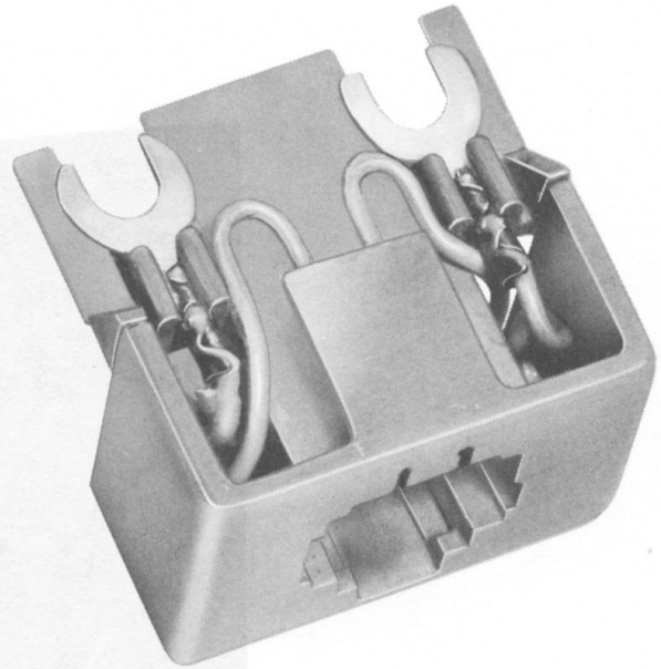
Fig. 24—248A Adapter
