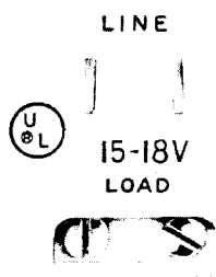
Fig. 5—2012B Transformer
