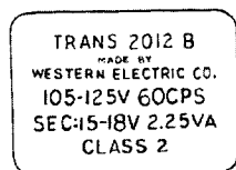
Fig. 5—2012B Transformer
