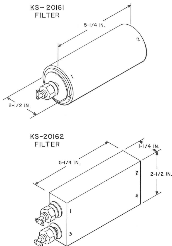
Fig. 1—KS-Type Filters
