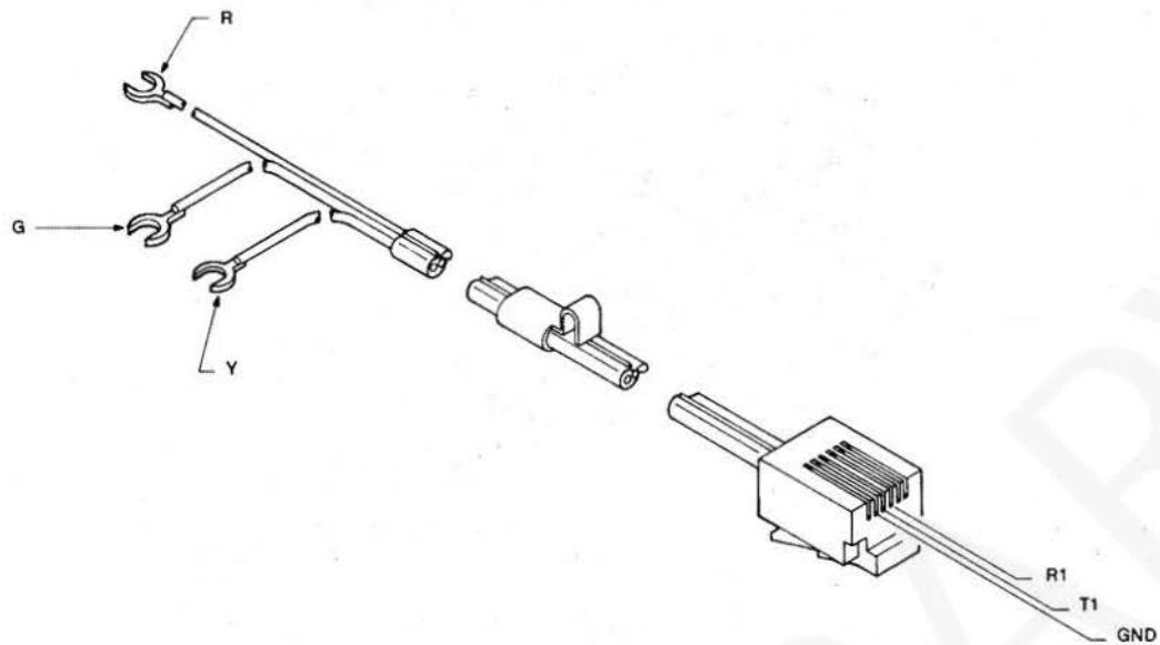
Fig. 6 - NE-D3QA Cord
