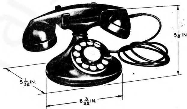
FIG. 2—202-TYPE DIAL
