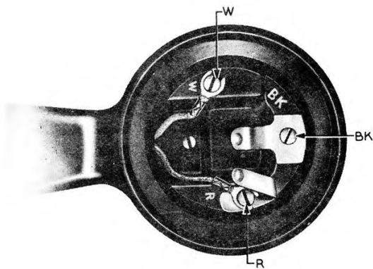
FIG. 3—F4-TYPE HANDSET
