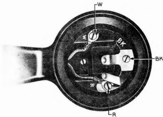
FIG. 3—F4-TYPE HANDSET
