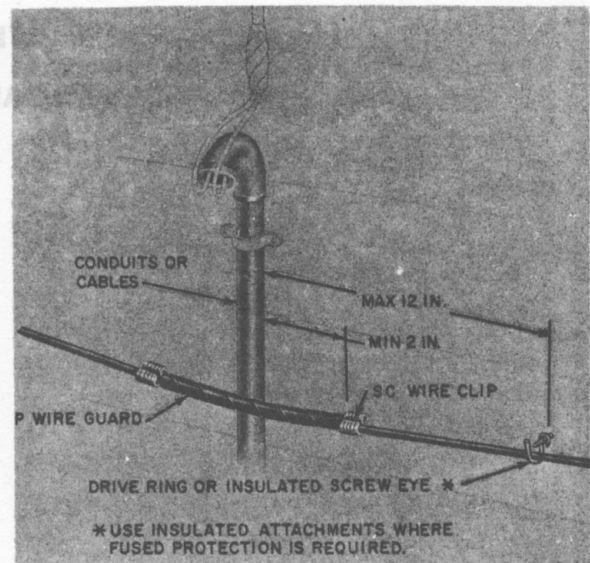
Fig. 13—Drop Wire Crossing Over Conduit
