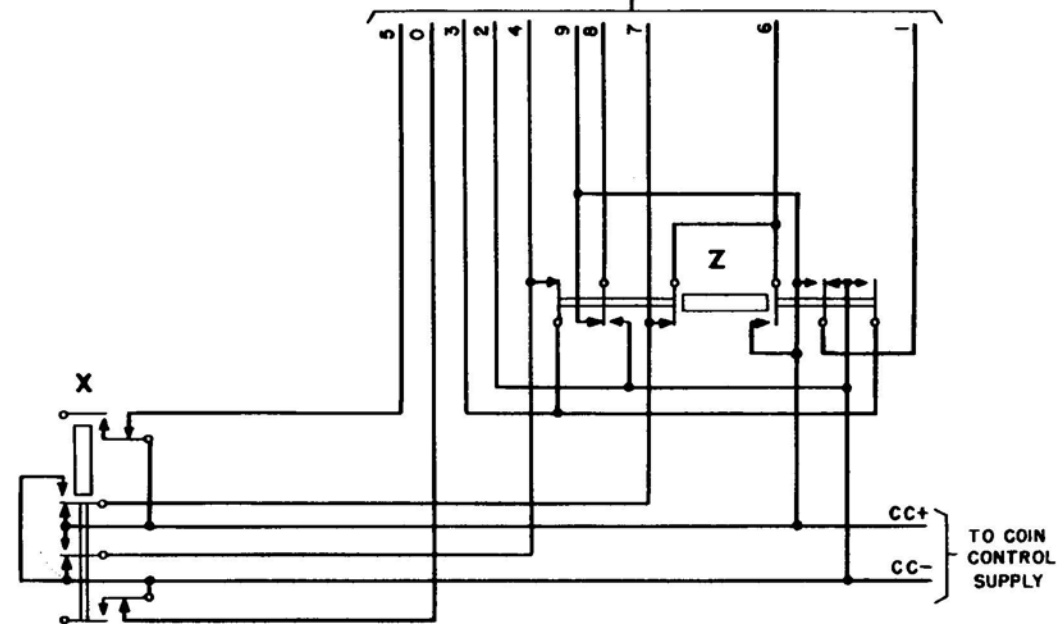
FIG. 6 DIGIT CODING
